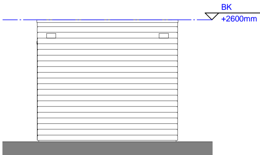
Achteraanzicht
